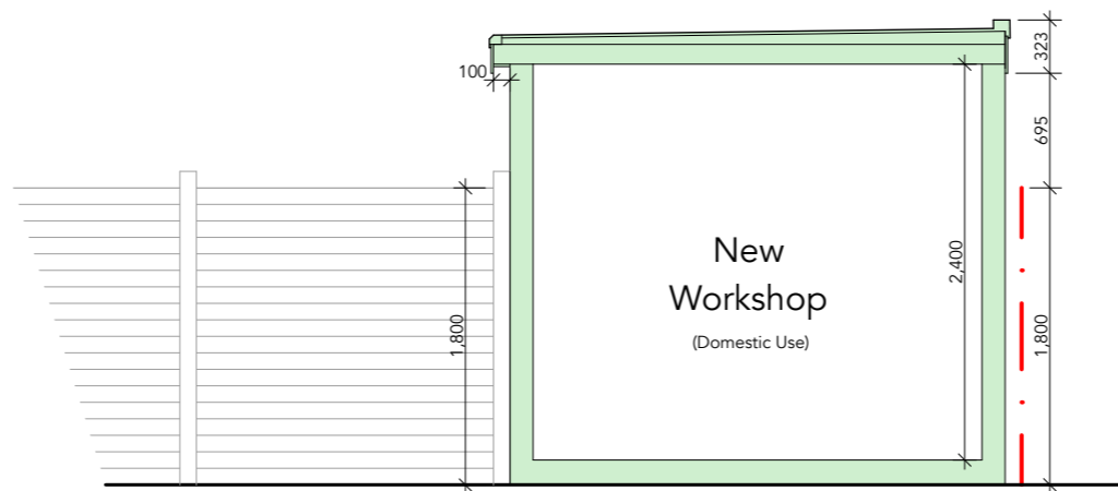
Section C-C Scale:- 1:50
