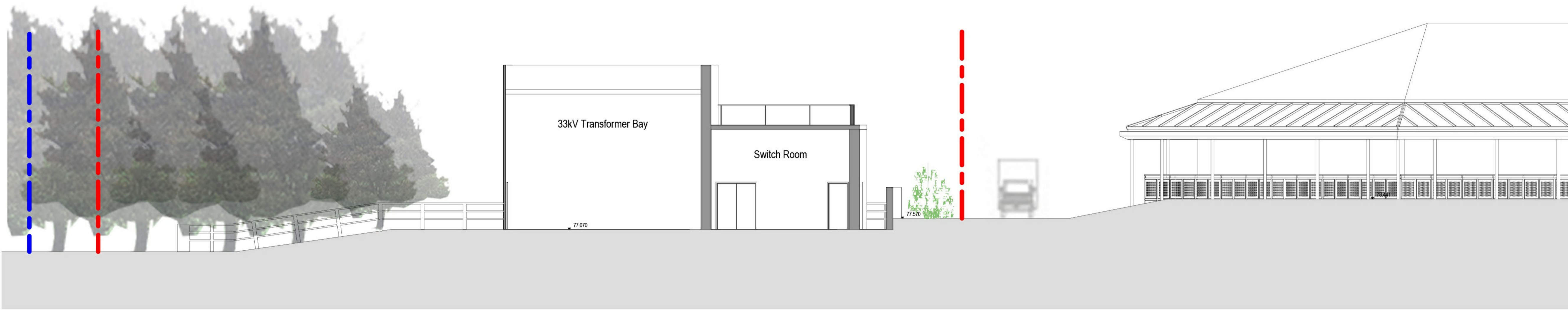
1 Site Section Substation (GEL) 1 : 100
